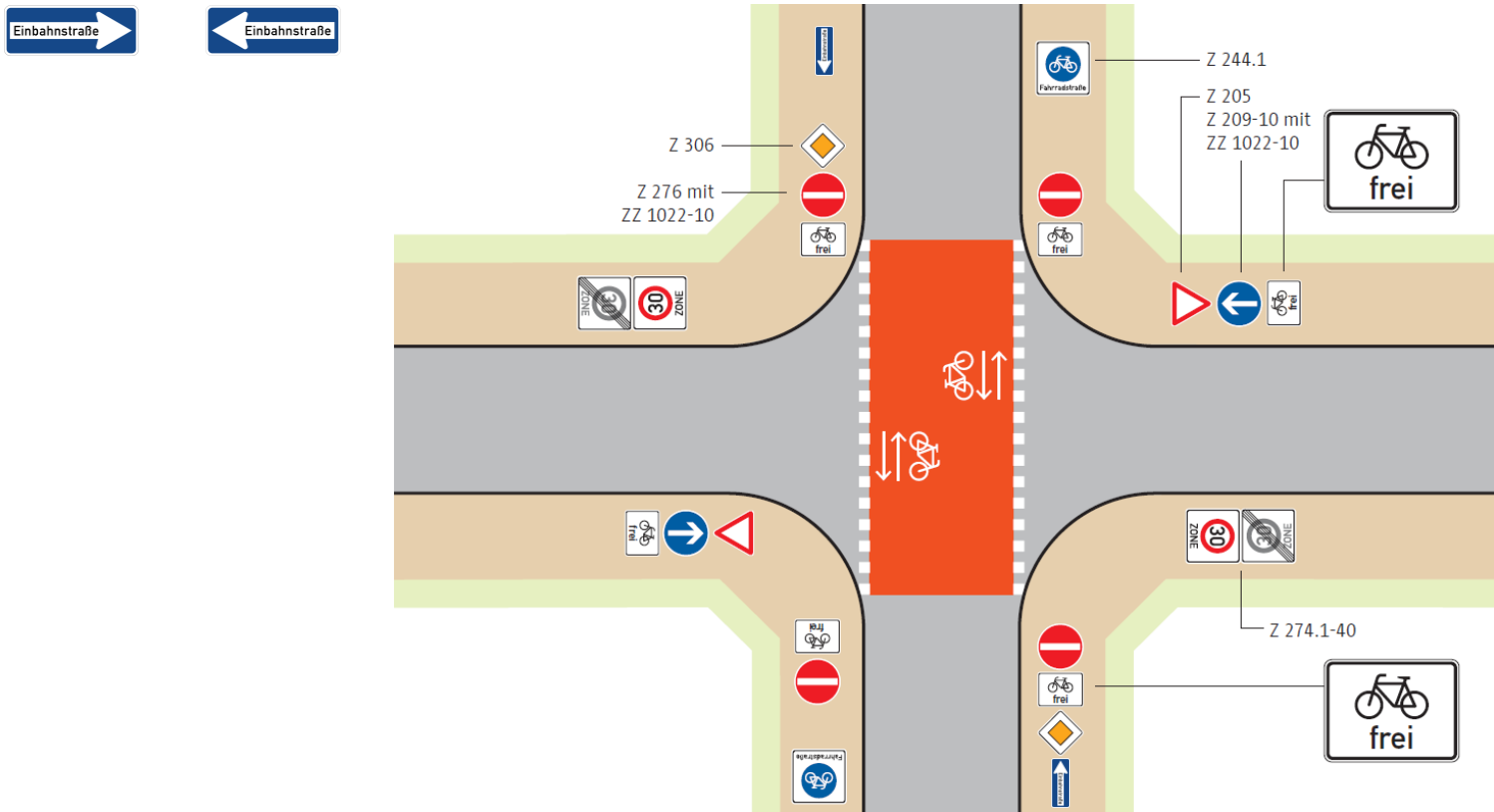
Abbildung 1: Modalfilter mit Verkehrszeichen (gegenläufige Einbahnstraße)
